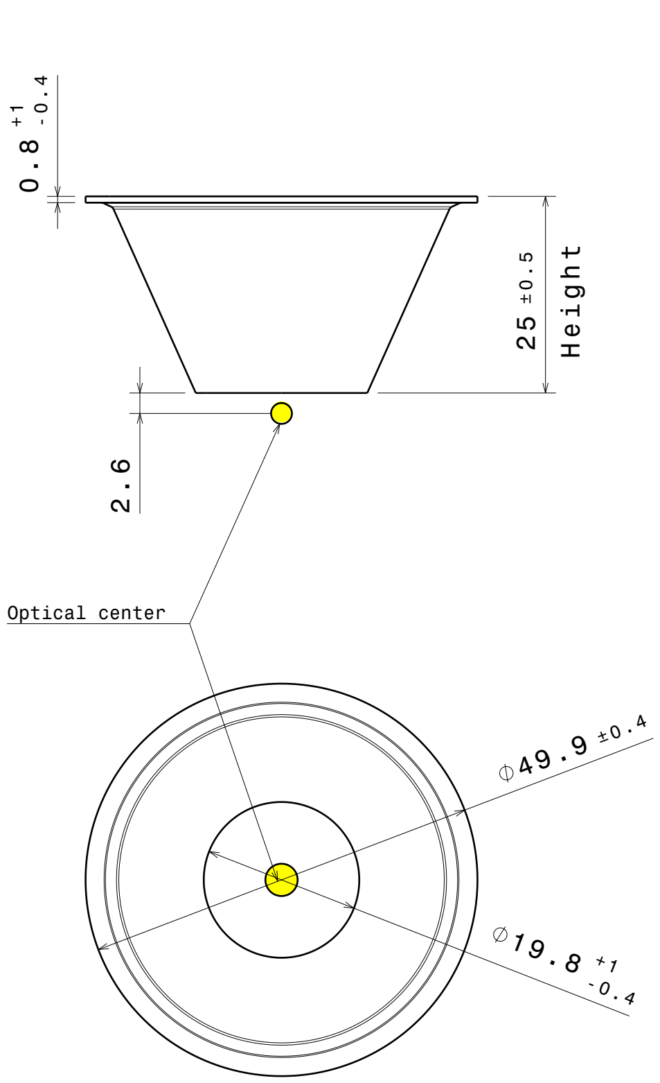
Top view Scale: 3:2
