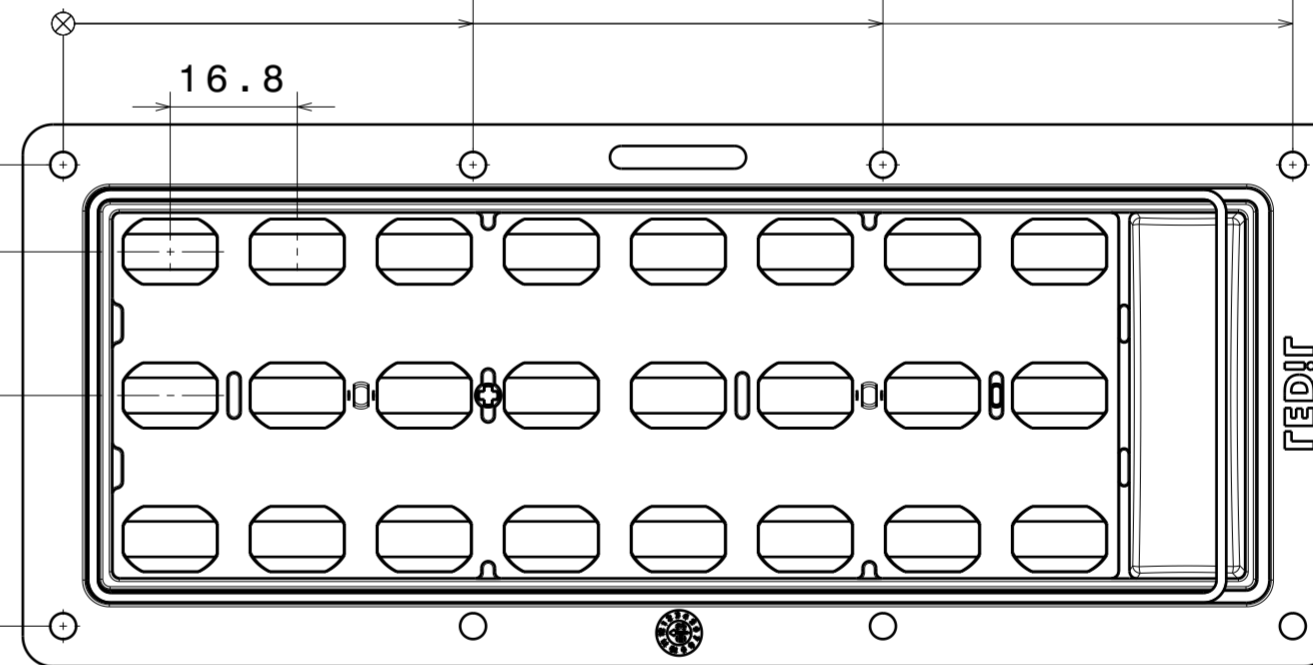
Rear view Scale: 1:1
