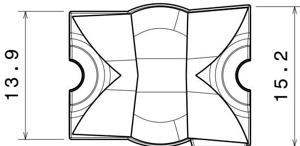
Top view Scale: 5:2
