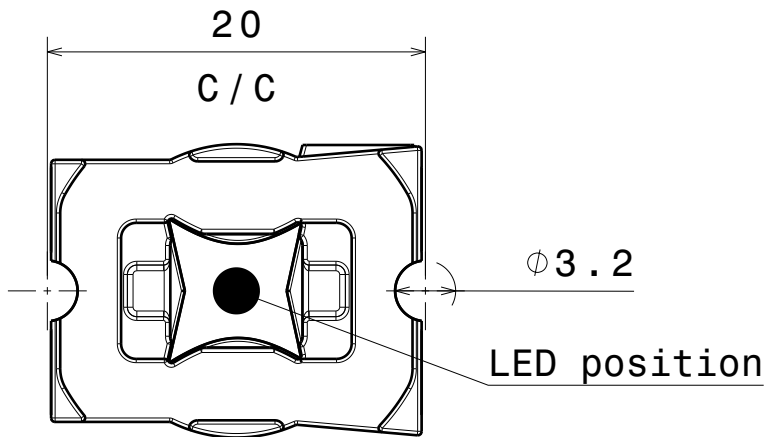
Bottom view Scale: 5:2
