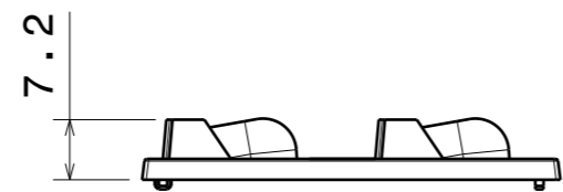
Scale: 1:1
