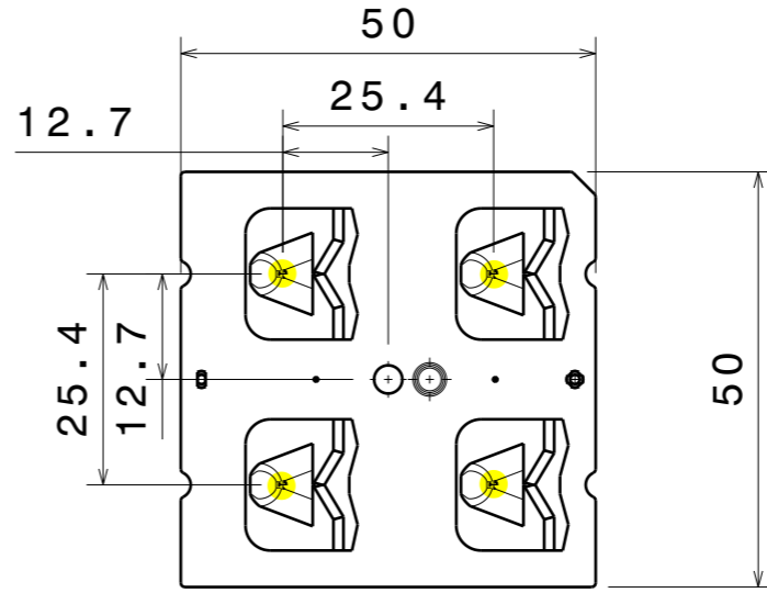
Scale: 1:1
