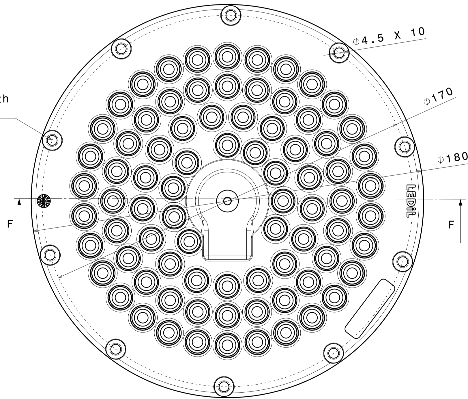
Top View Scale: 1:1
